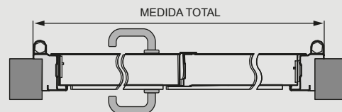
Puerta Turia EI2 30-60-90
